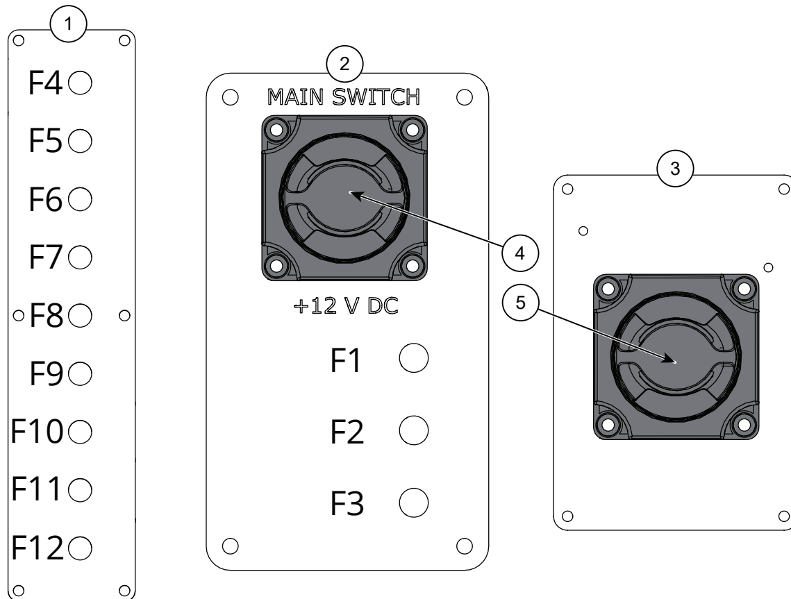
Kuva 8.1 Buster XL/XXL:n päävirtakytkimet ja sulakepaneelit
