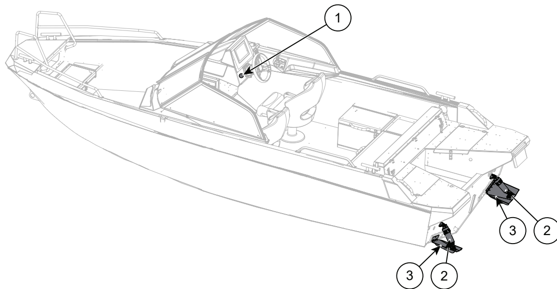
Kuva 5.4 Buster XL/XXL:n trimmijärjestelmän komponentit
