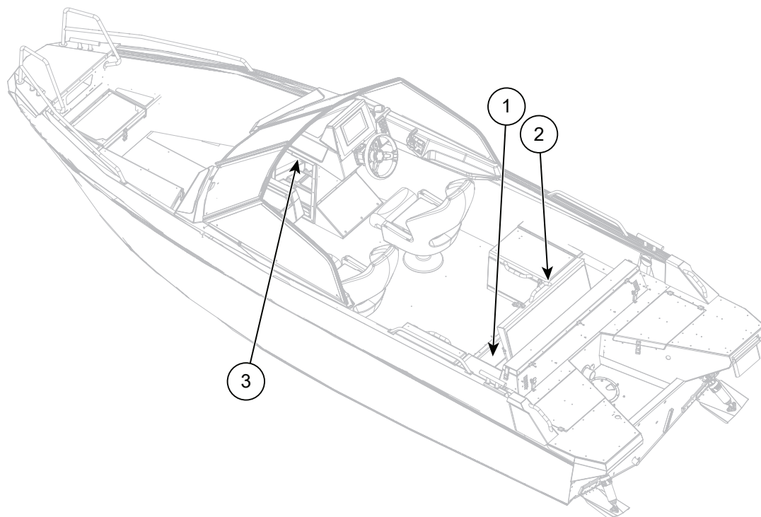
Kuva 8.2 Buster XL/XXL:n sulakepaneelin sijainnit
