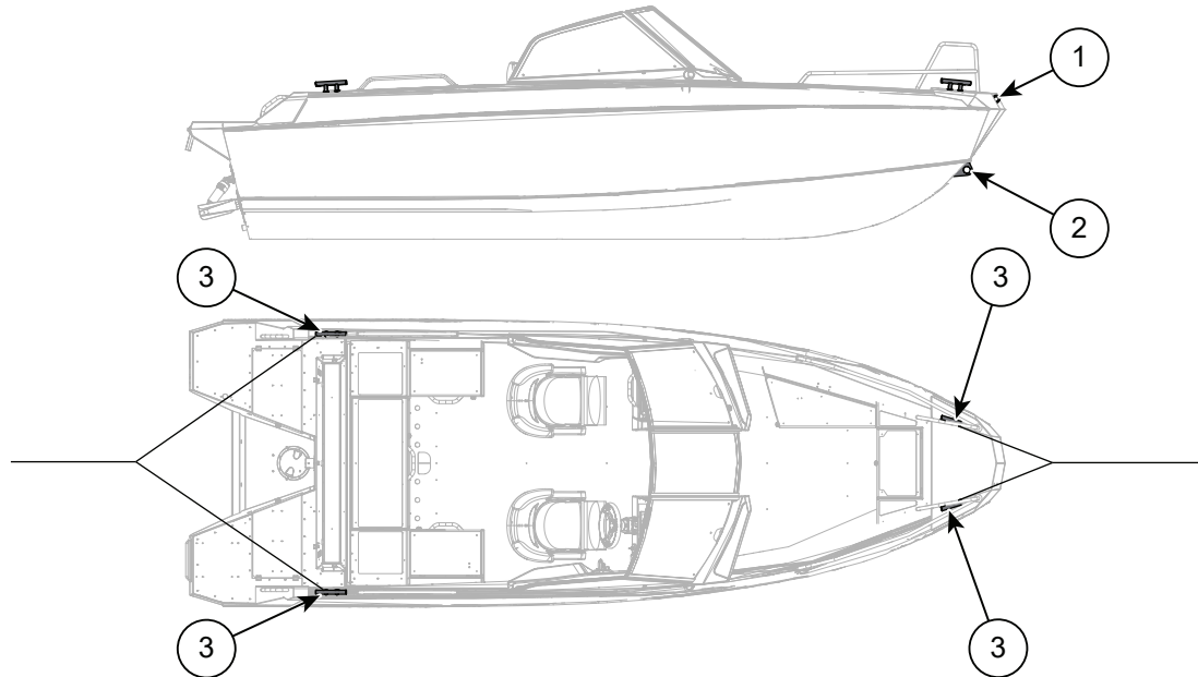
Kuva 5.5 Buster XL/XXL:n kiinnitys- ja hinauspisteet
