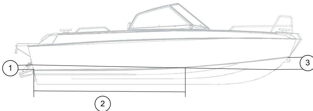
Kuva 3.1 Buster XL/XXL:n anti-fouling-maalialue
