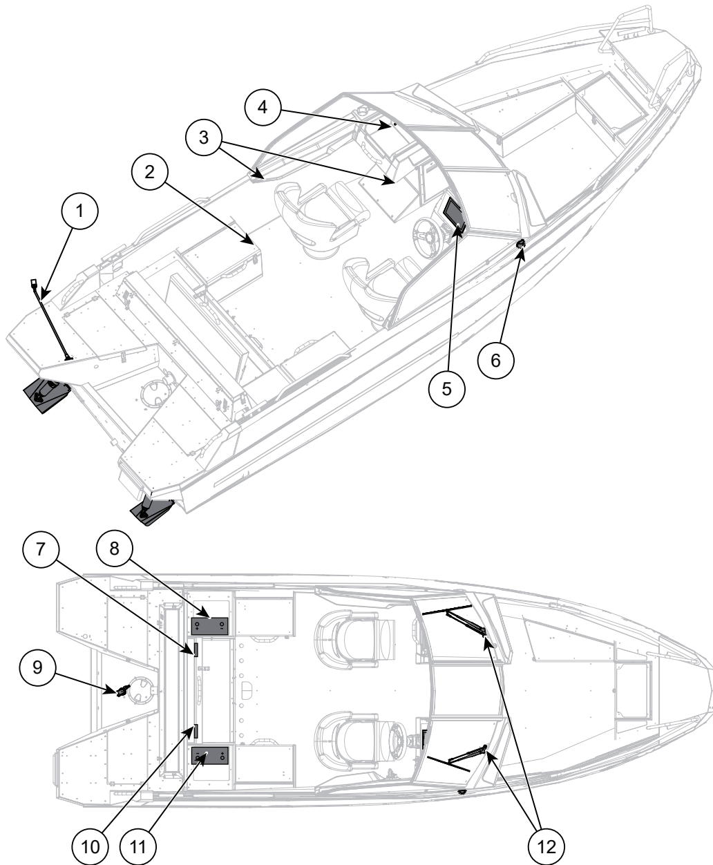
Kuva 8.3 Buster XL/XXL:n sähkölaitteet
