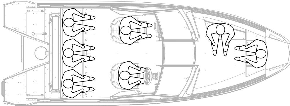
Kuva 4.1 Buster XL:n istuimet enintään seitsemälle (7) matkustajalle
