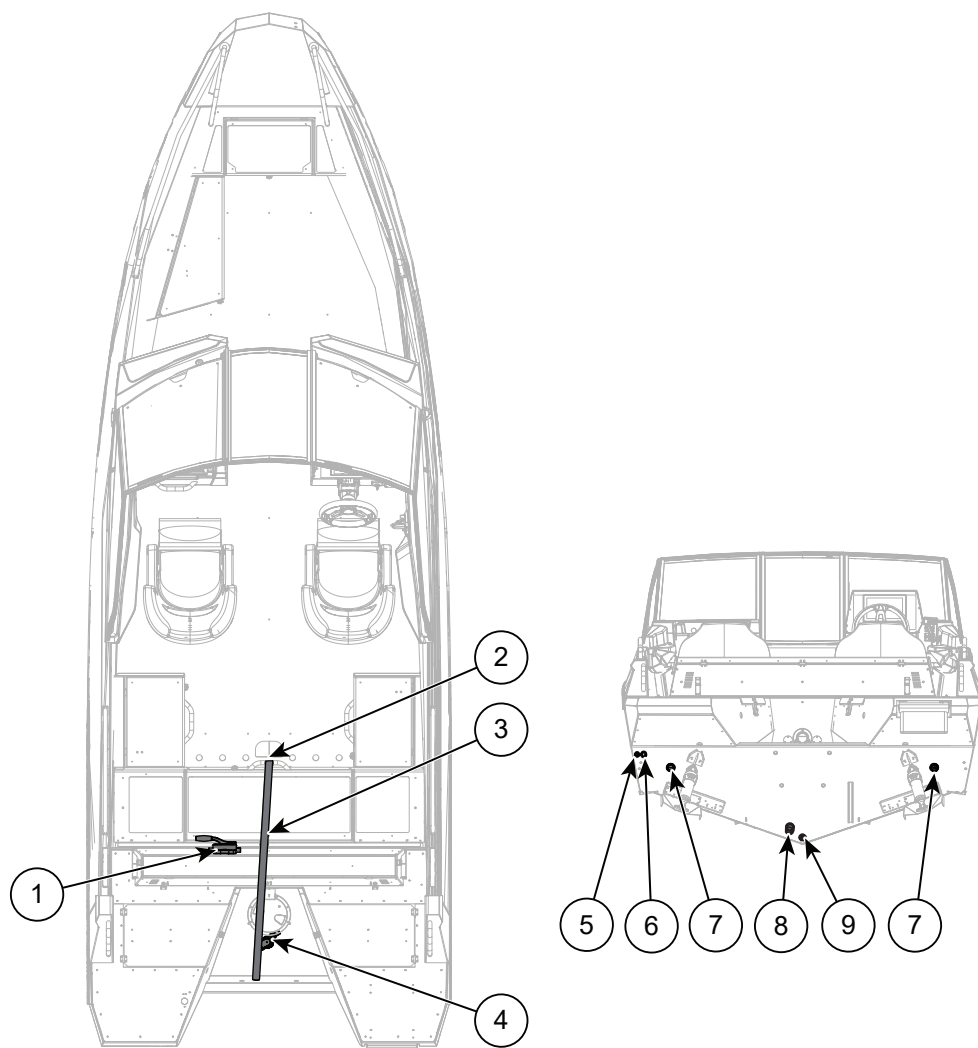
Kuva 9.1 Buster XL/XXL:n tyhjennysvarustus
