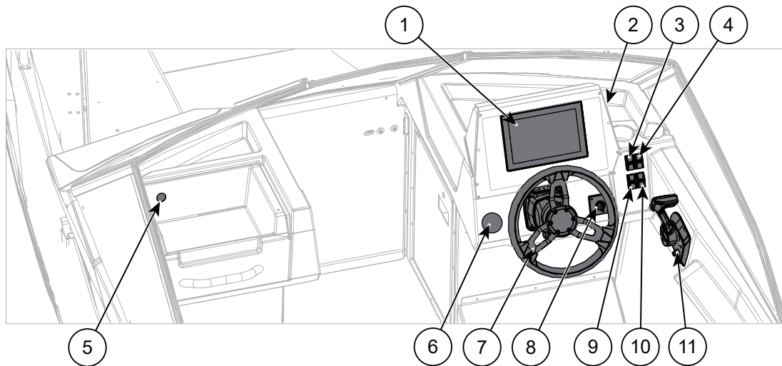
Kuva 5.1 Buster XL/XXL:n ohjauspisteen hallintalaitteet
